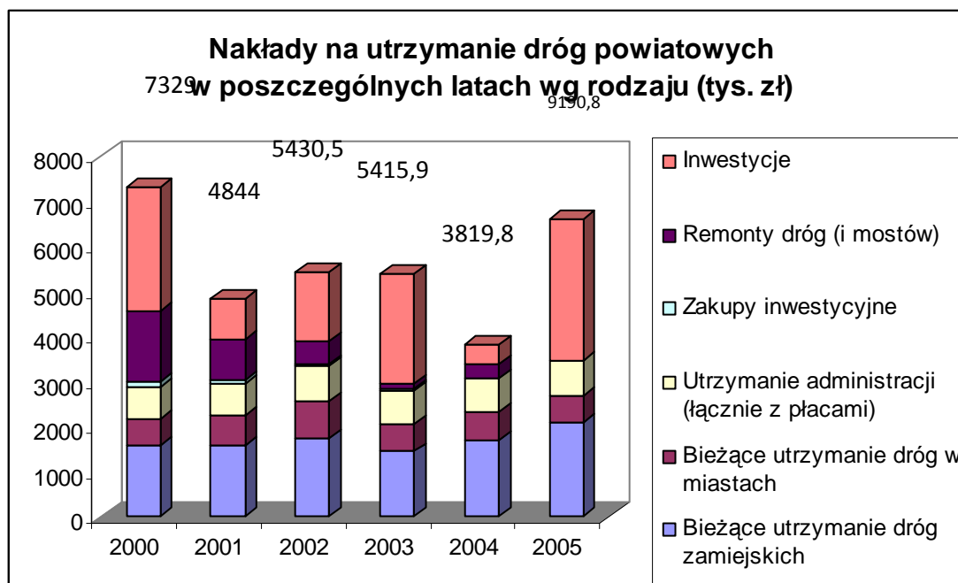
Wykres 29. Nakłady na utrzymanie dróg powiatowych wg rodzaju w latach 2000-2005.
