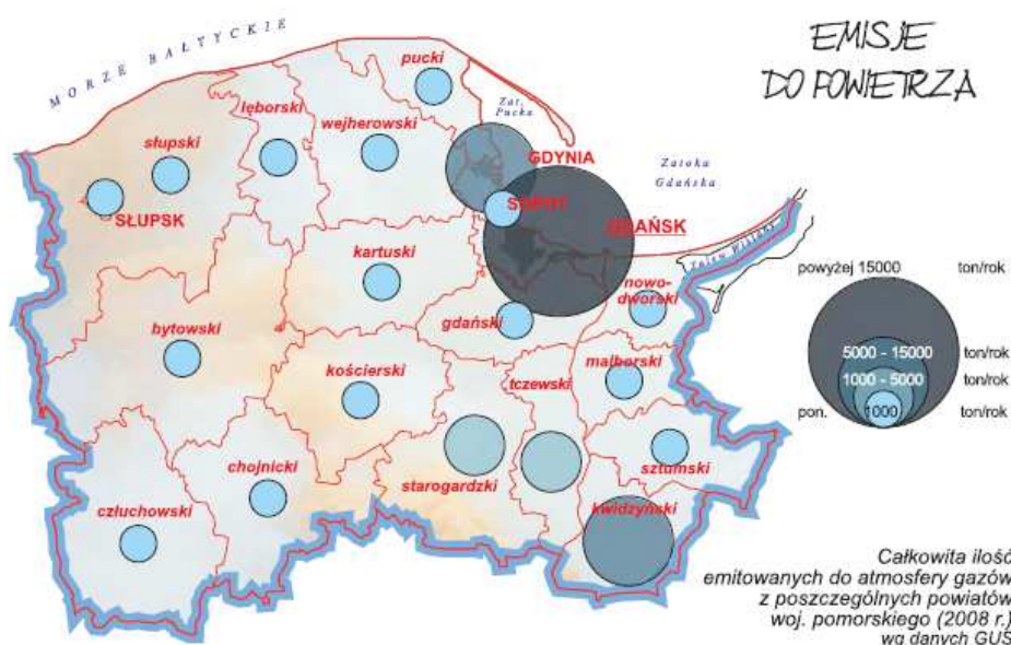
Mapa 21. Całkowita ilość emitowanych do atmosfery gazów z poszczególnych powiatów województwa pomorskiego.
